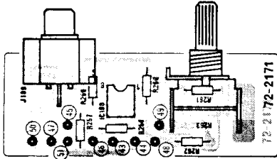
OUTPUT AMP. PCB
